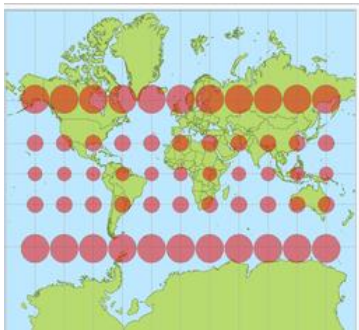
Меркатор проекциясындағы аудандардың бұрмаланулары
